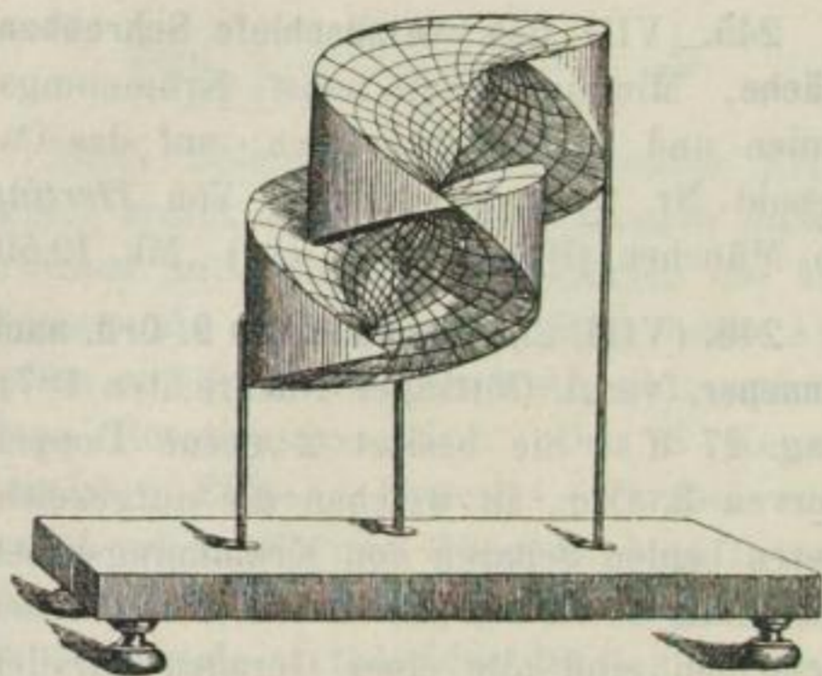
248. (XVII, 1.) Minimalfläche, welche eine Schar reeller Parabeln enthält, deren Ebenen mit einer festen Ebene des Raumes einen constanten Winkel einschliessen.
